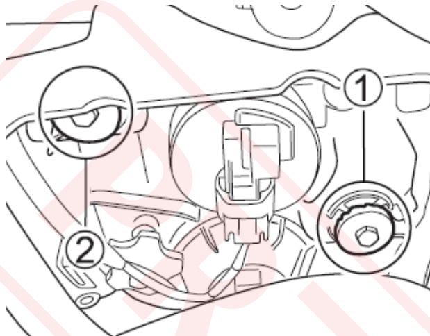
Światło mijania
